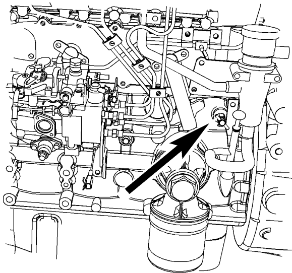
Рисунок 1 Кран для слива охлаждающей жидкости
